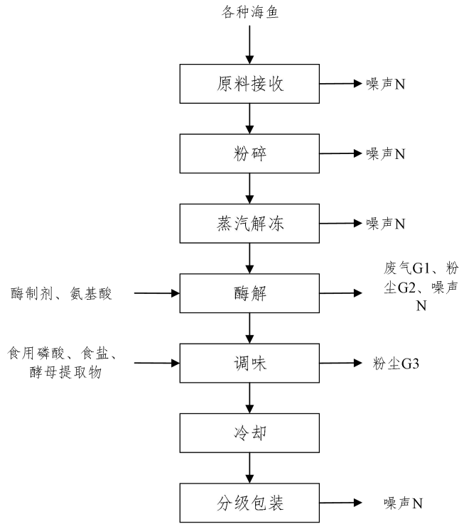
图3.3-2 鱼蛋白生产工艺及产污节点图
