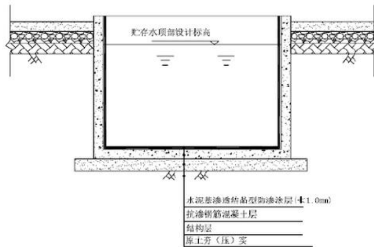
图 6.5-1 污水设施防渗层示意图
