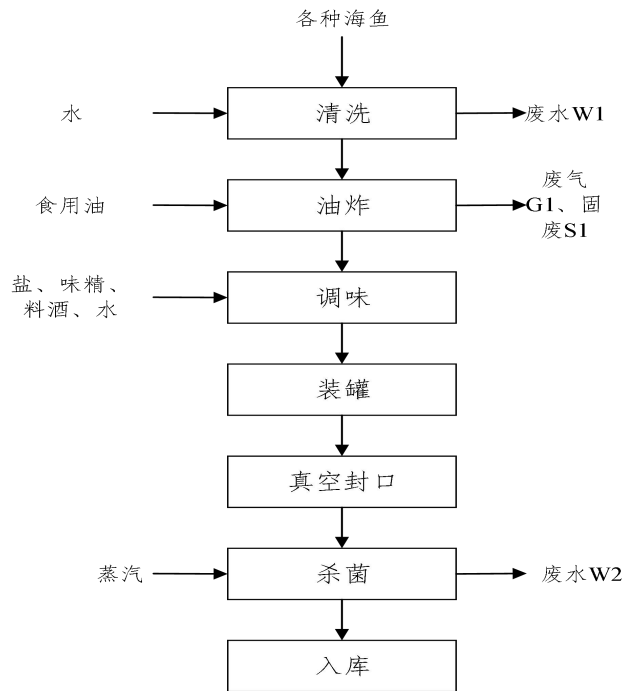
图3.3-3 即食食品生产工艺及产污节点图
