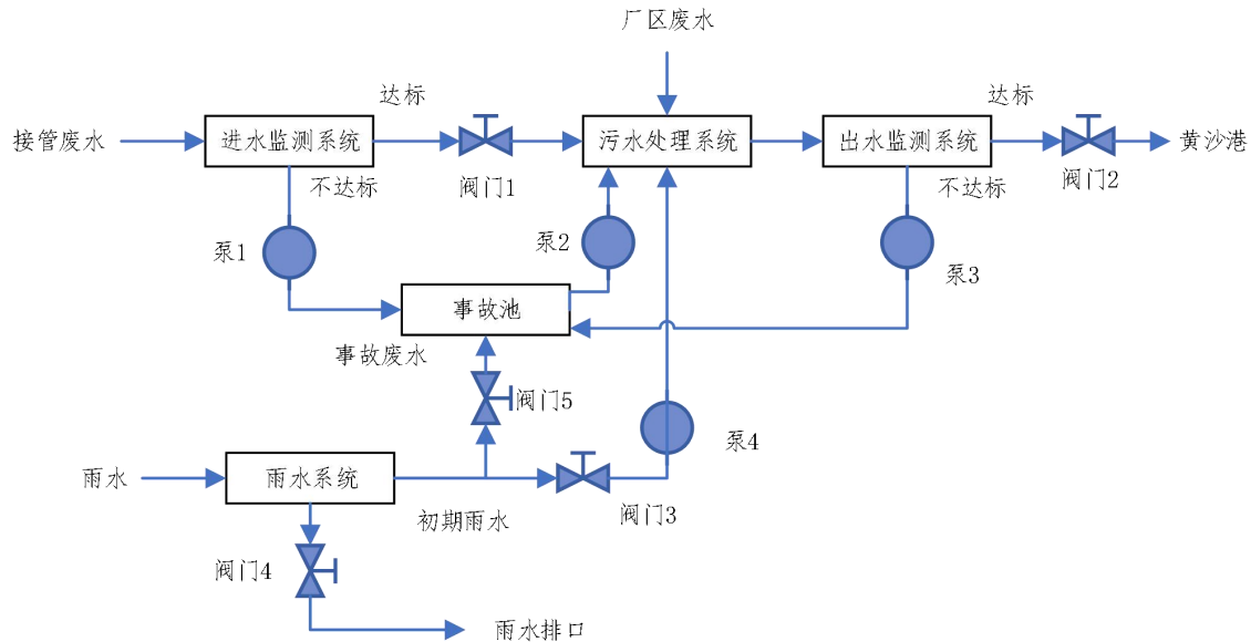
图6.7-1 防止事故水进入外环境的控制、封堵系统图
