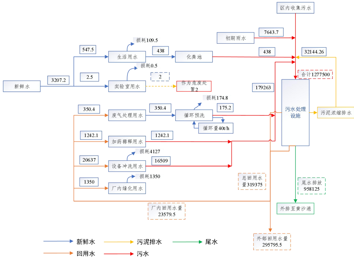
图 3.7-1 污水处理厂一期工程水平衡图
