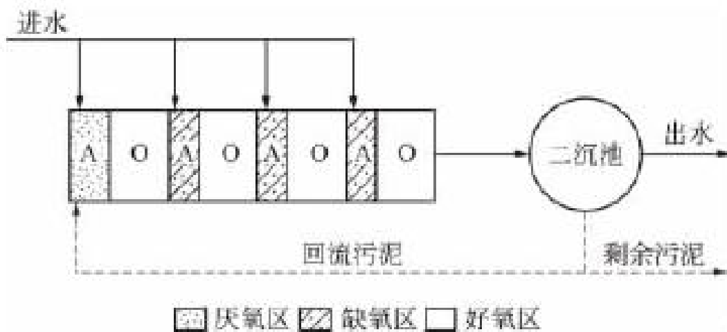
图 3.4-6 多级 AO 工艺流程图
