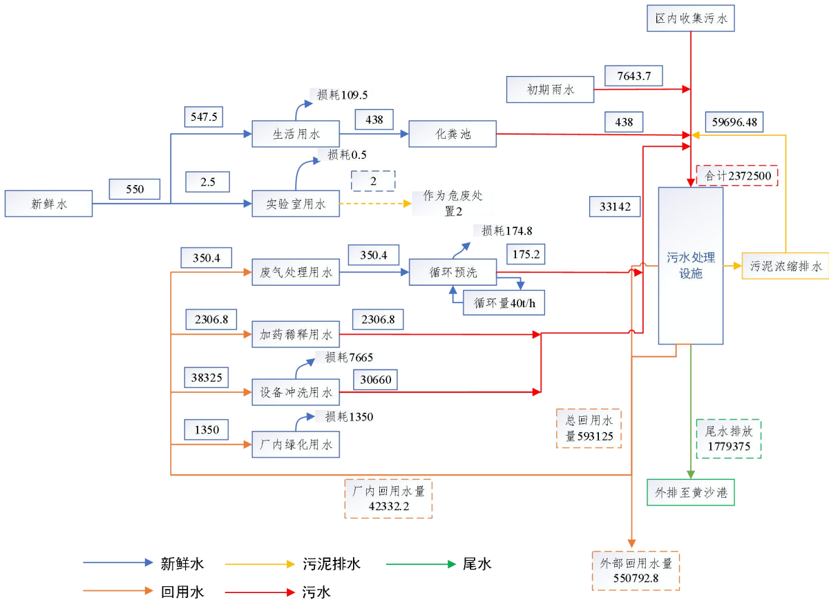
图 3.7-2 污水处理厂全厂水平衡图
