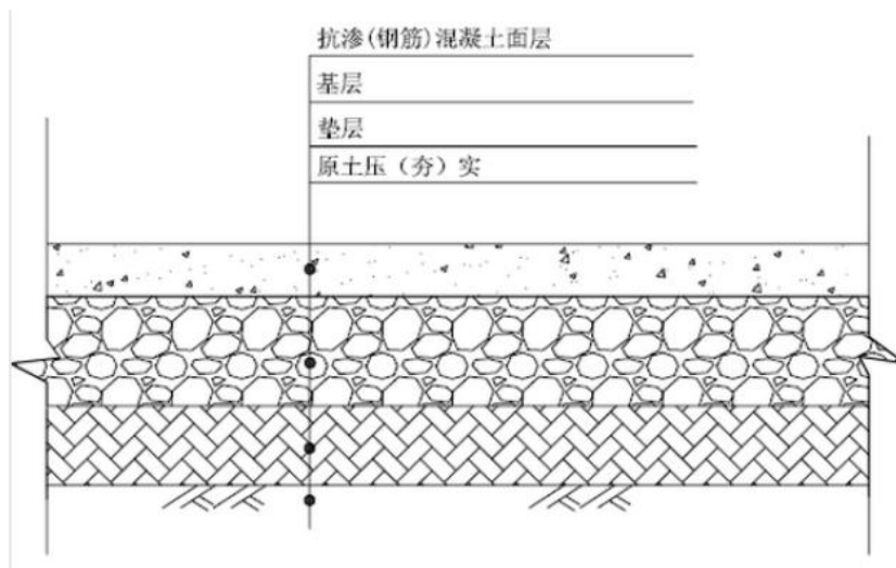
图 6.5-2 一般污染防治区典型防渗结构示意图
