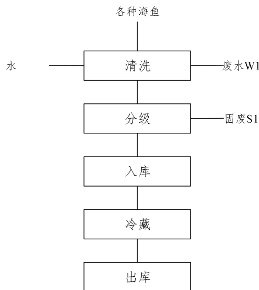
图3.3-4 鱼产品冷链物流工艺及产污节点图
