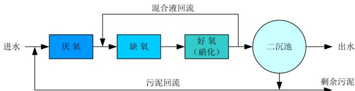
图 3.4-1 传统 A/A/O 工艺流程图
