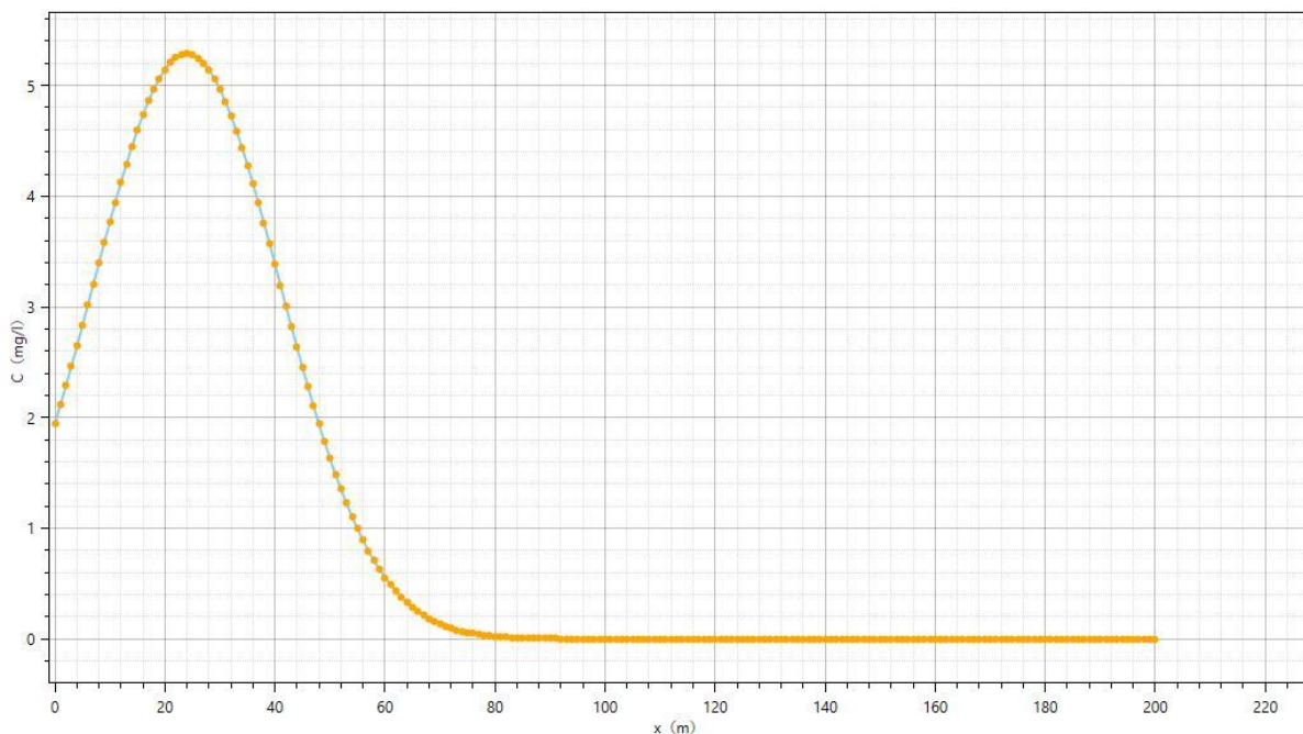
图 5.6-4 下游轴向 CODMn 浓度随时间变化曲线（7200d）
