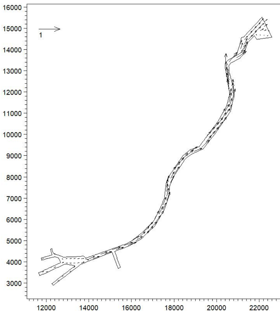
图 5.2-6 枯水期排污口附近落急时刻流场 (m)
