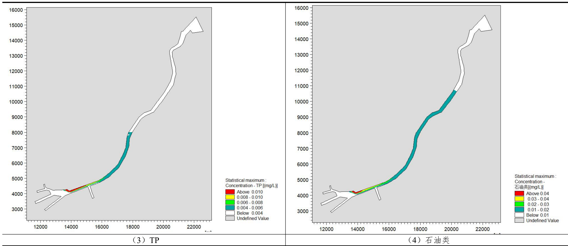
图 5.2-8 工况 2 各特征污染物浓度增量包络线图
