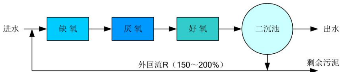
图 3.4-2 倒置 A/A/O 工艺流程图
