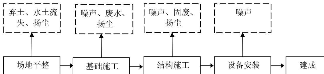
图 3.6-1 污水处理厂施工工艺流程图
