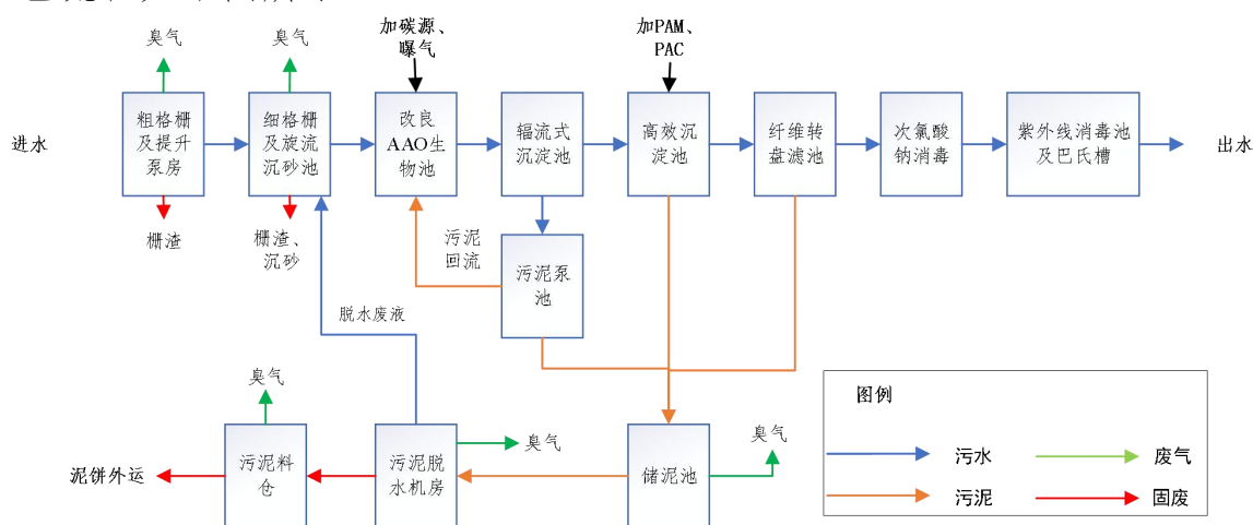
图 3.5-1 污水处理工艺流程图
