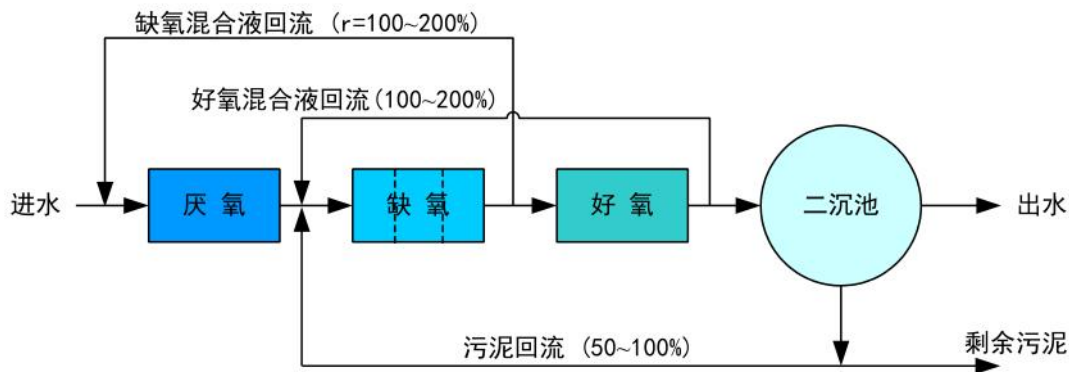
图 3.4-5 UCT（VIP）A/A/O 工艺工程实例图
