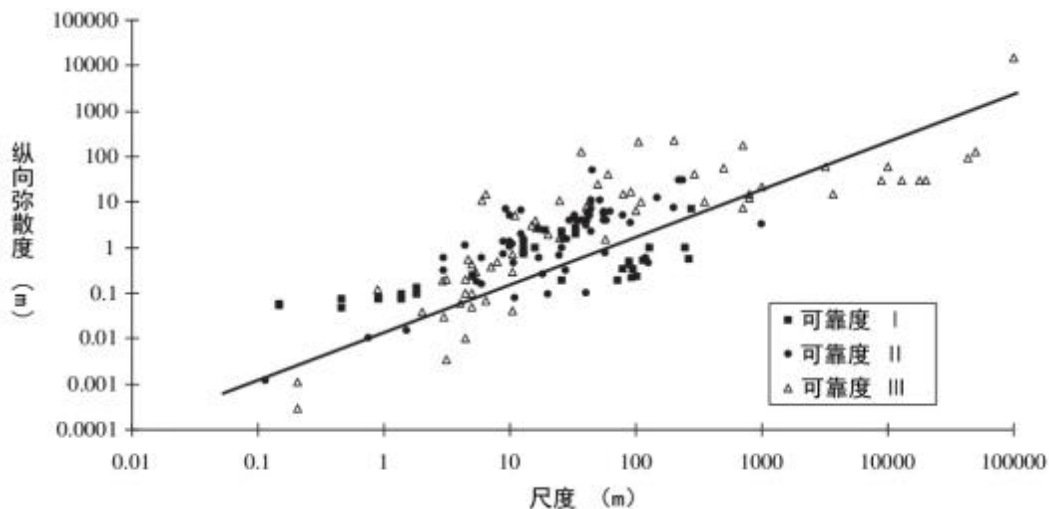
图 5.6-1 纵向弥散度与观测尺度之间的关系
