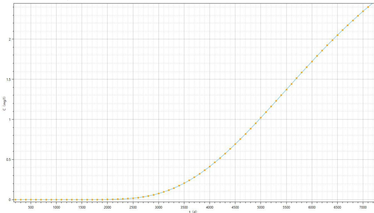
图 5.6-2 东侧厂界 \text{COD}_{\text{Mn}} 浓度随时间变化曲线（ x=100 ， y=10 ）
