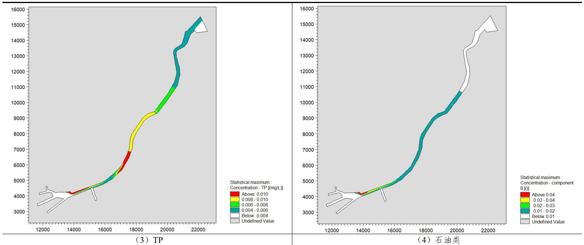
图 5.2-10 工况 4 各特征污染物浓度增量包络线图
