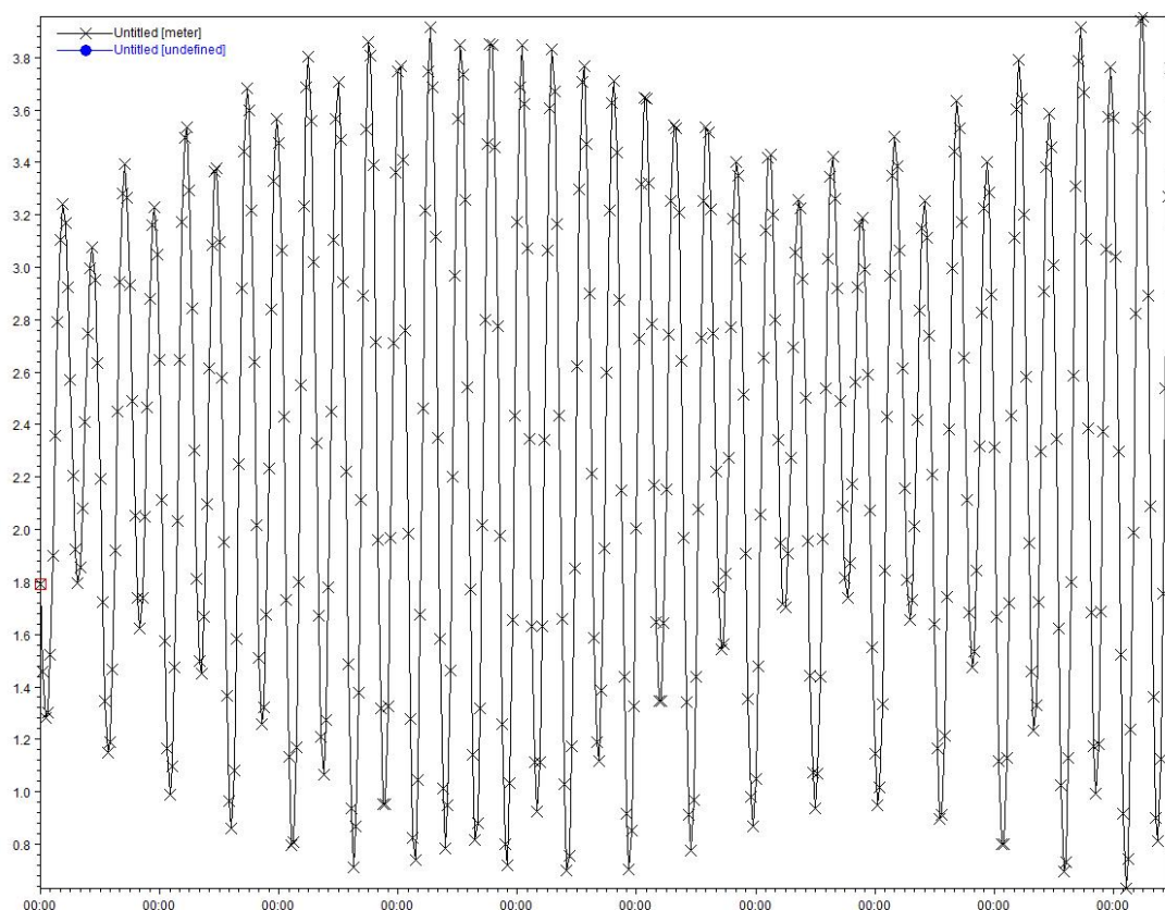
图 5.2-4 海域潮位过程
