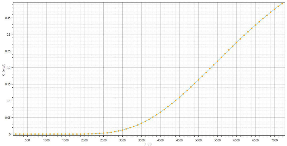
图 5.6-5 东侧厂界 \text{NH}_3\text{-N} 浓度随时间变化曲线（ x=100 ， y=10 ）
