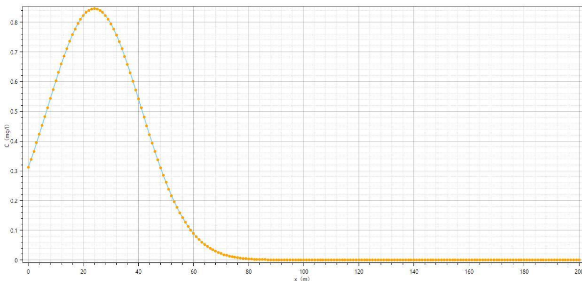
图 5.6-7 下游轴向 \text{NH}_3\text{-N} 浓度随时间变化曲线 (7200d)
