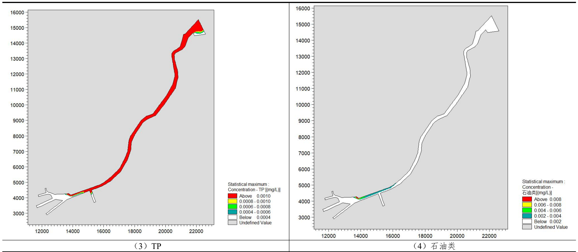
图 5.2-9 工况 3 各特征污染物浓度增量包络线图 (m)
