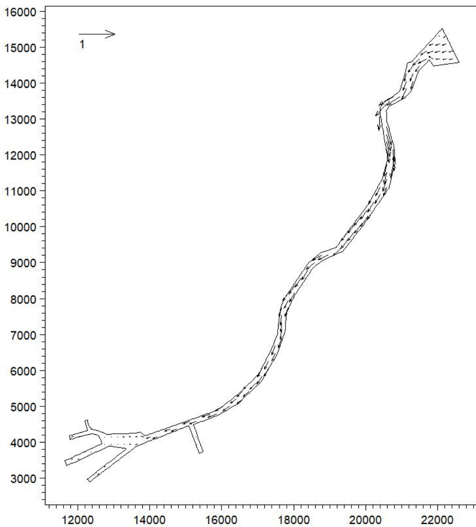
图 5.2-5 枯水期排污口附近涨急时刻流场 (m)
