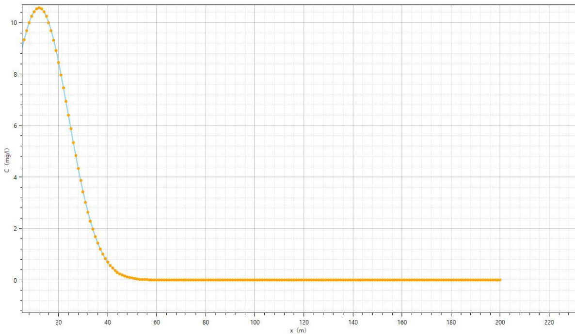
图 5.6-3 下游轴向 CODMn 浓度随时间变化曲线（3600d）
