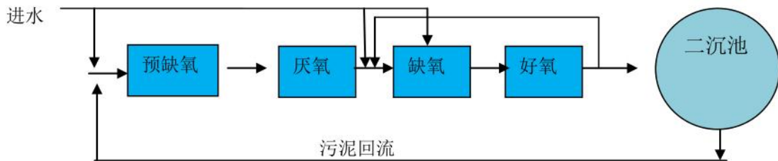
图 3.4-3 改良型 A/A/O 工艺流程图
